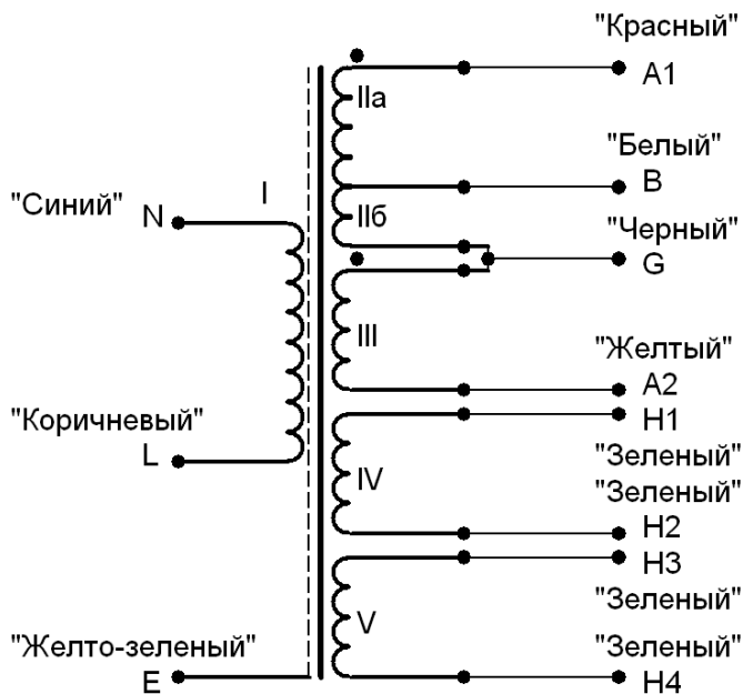
Рис1. Схема трансформатора.
