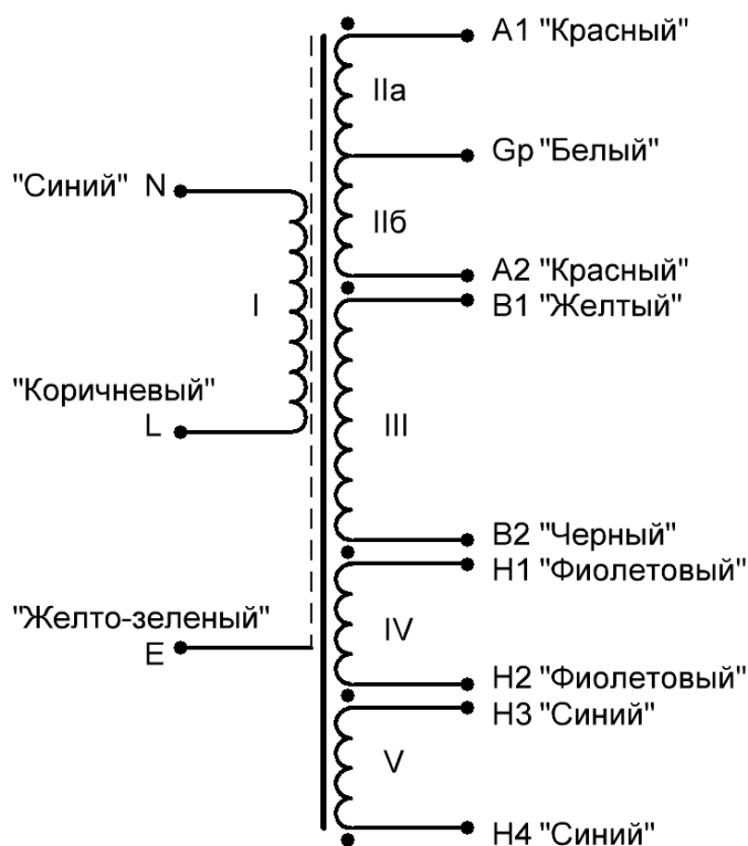
Рис.1 Схема трансформатора.
