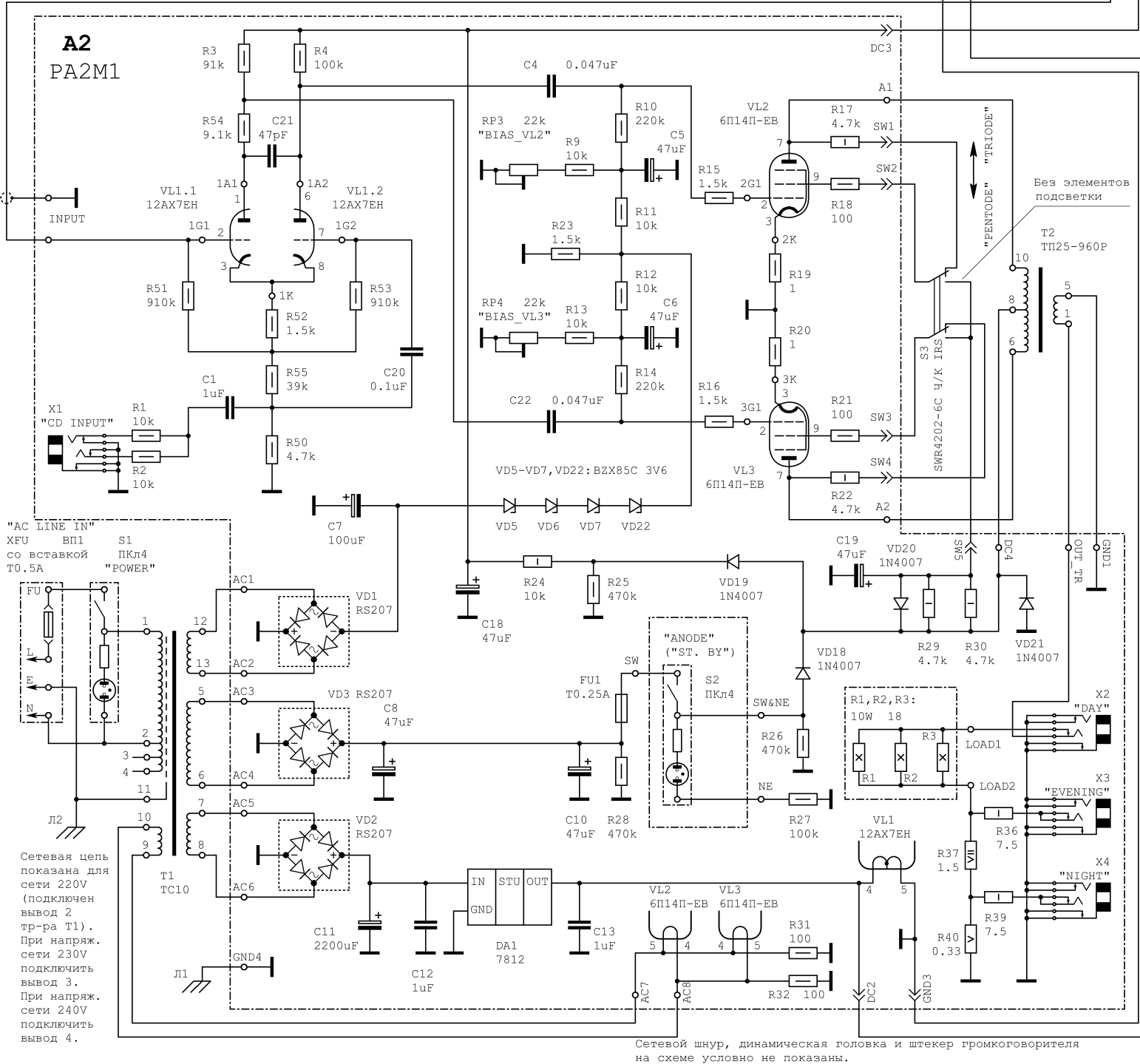
Goblin 10. Схема электрическая принципиальная.
